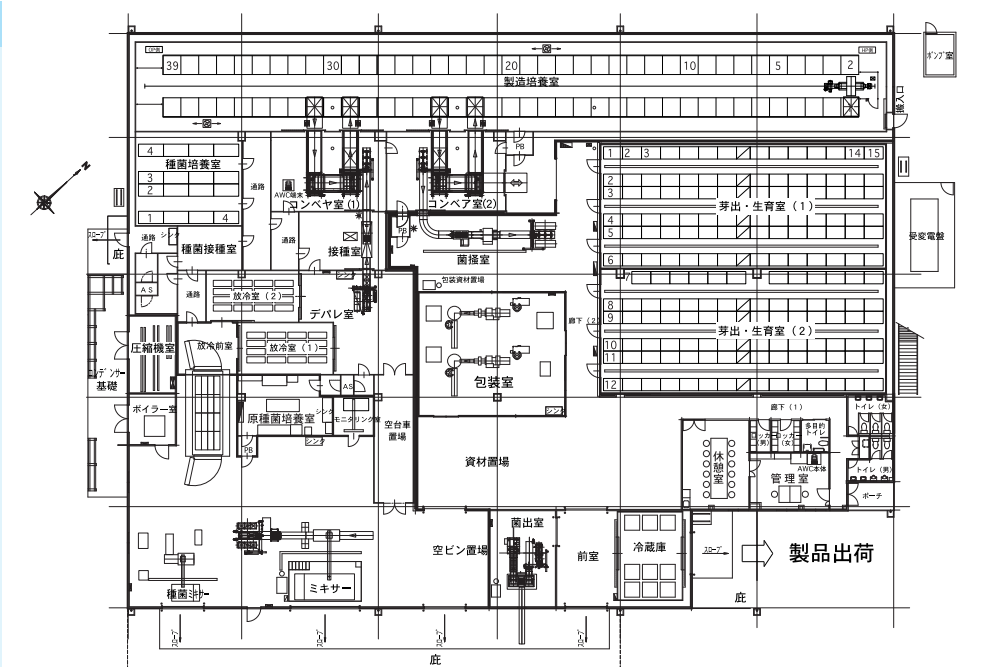
* 施設平面図 *
