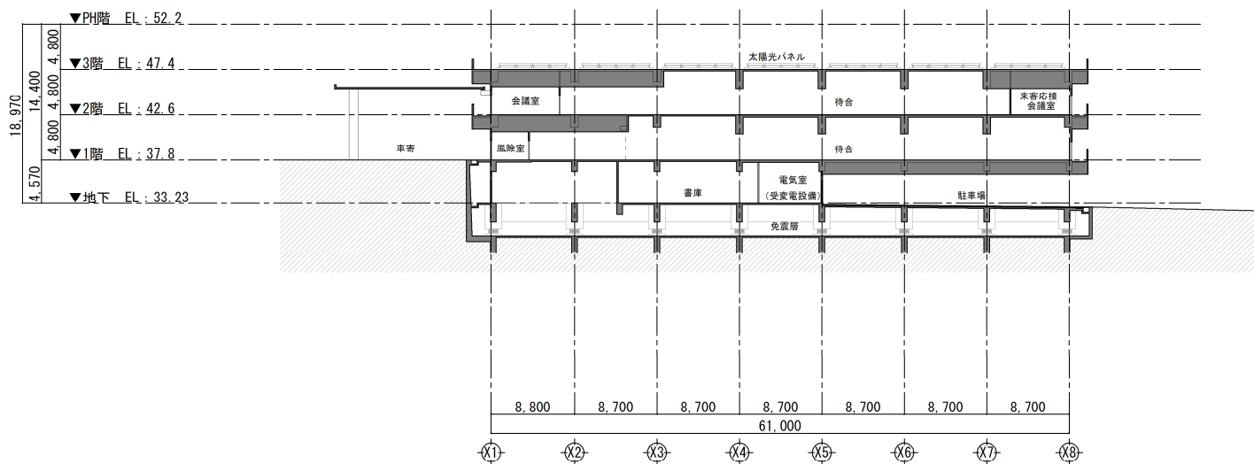
B断面図 S=1/500
