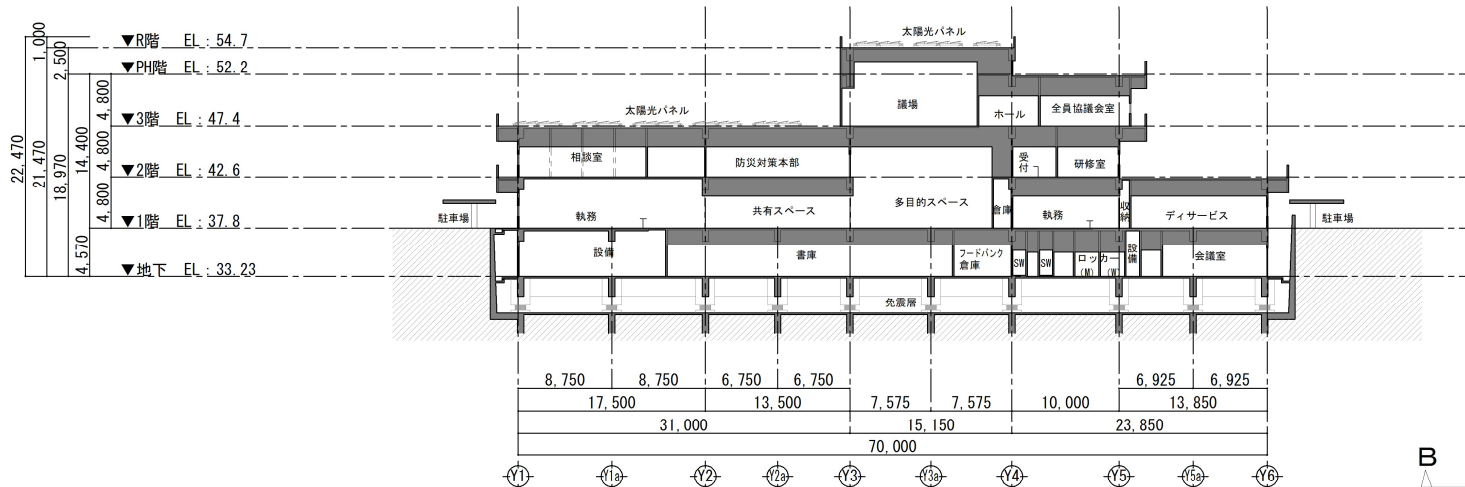
A断面図 S=1/500
