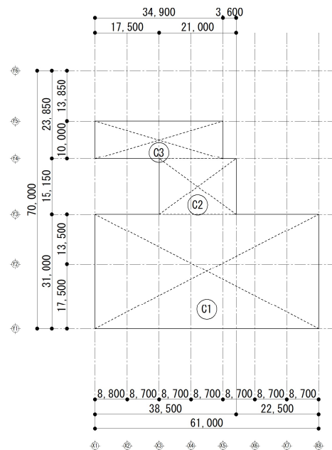
2階求積図
