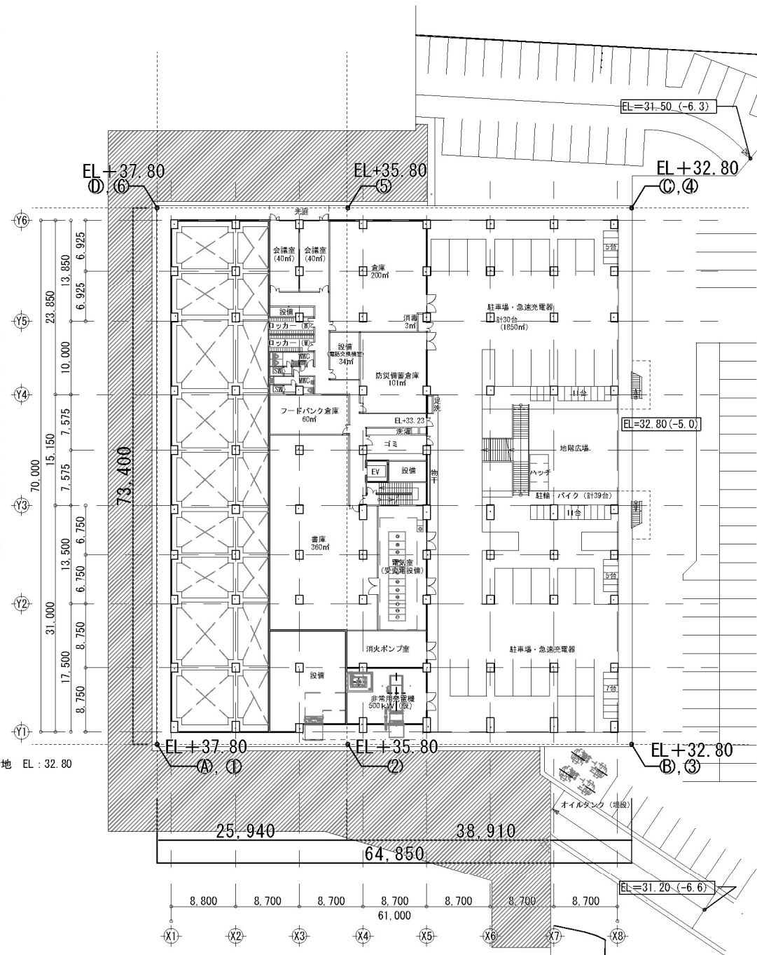
地下平面図 S=1/500
