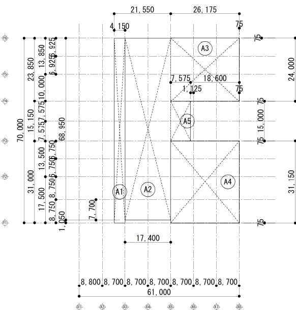
地下求積図
